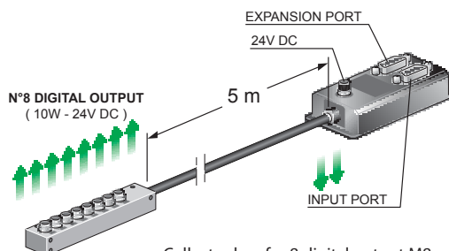
Collector box for 8 digital output M8 connection Box distribuzione 8 output digitali con connessioni M8
